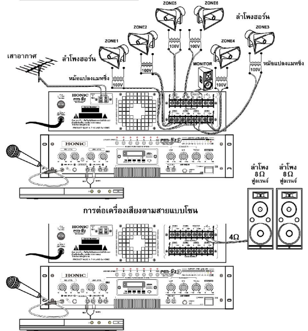
การต่อเครื่องเสียงทั่วไป แบบระบบลำโพงตู้ ภายในอาคาร และนอกอาคาร
